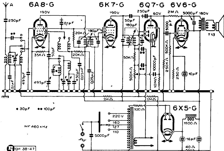
WATT RADIO - MOD. «AUREA PICCOLO» 1948 »
