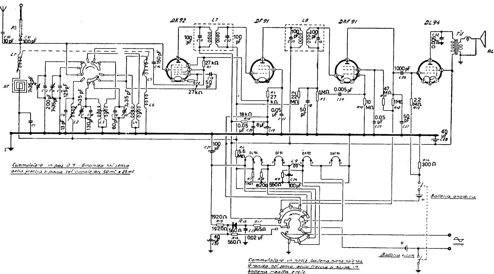
TELEFUNKEN (COMPAGNIA RADIORICEVITORI). Mod. CHERI T20. Apparecchio portatile alimentato a pile e adatto anche per alimentazione in alternata. Gamma onde medie e due bande allargate a 50 e a 25 metri. Commutatore a tre posizioni per funzionamento a potenza intera o ridotta, a pile e per funzionamento con la rete-luce. Media freq. 468 kc/s. Potenza d'usc. 0,2 watt.
