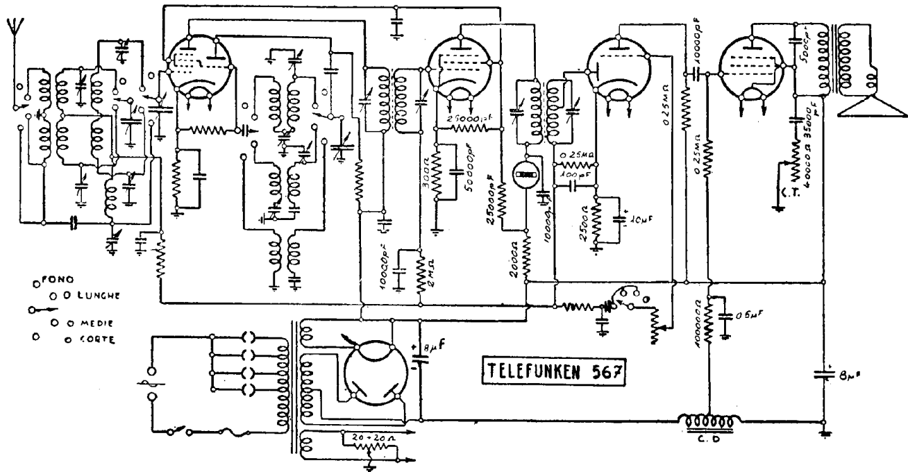
TELEFUNKEN RADIO (S. A. SIEMENS). — Mod. « 567 e 570 » anche « 576 e 577 », — Produzione 1936. — Media frequenza: 489 kHz. — Valvole: ACH1, RENS 1204, REN 924, RES 964 e RGN 1064.
