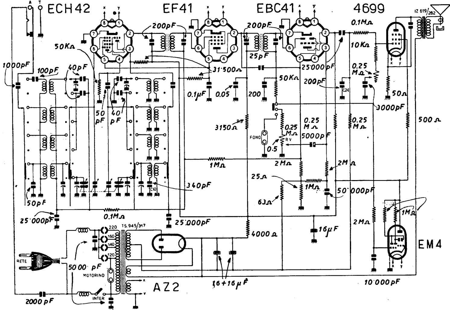
PHONOLA RADIO - Modd. 5512 A/B, 5517 A e 5518 - Medie divise e cinque bande onde corte. 5512 B radiofonografo: 5518 altoparlante M 201. MF a 470 kc. Placca finale 270 V, schermo 250 V. Altre placche 250 V, schermi 90 V. Uscita 6 W.
