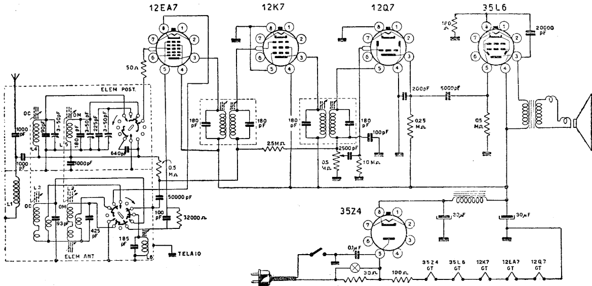
Fig. 8.6. - Supereterodina senza trasformatore di alimentazione, CA/CC. (Marelli mod. 9U65). V. fig. 8.5.
