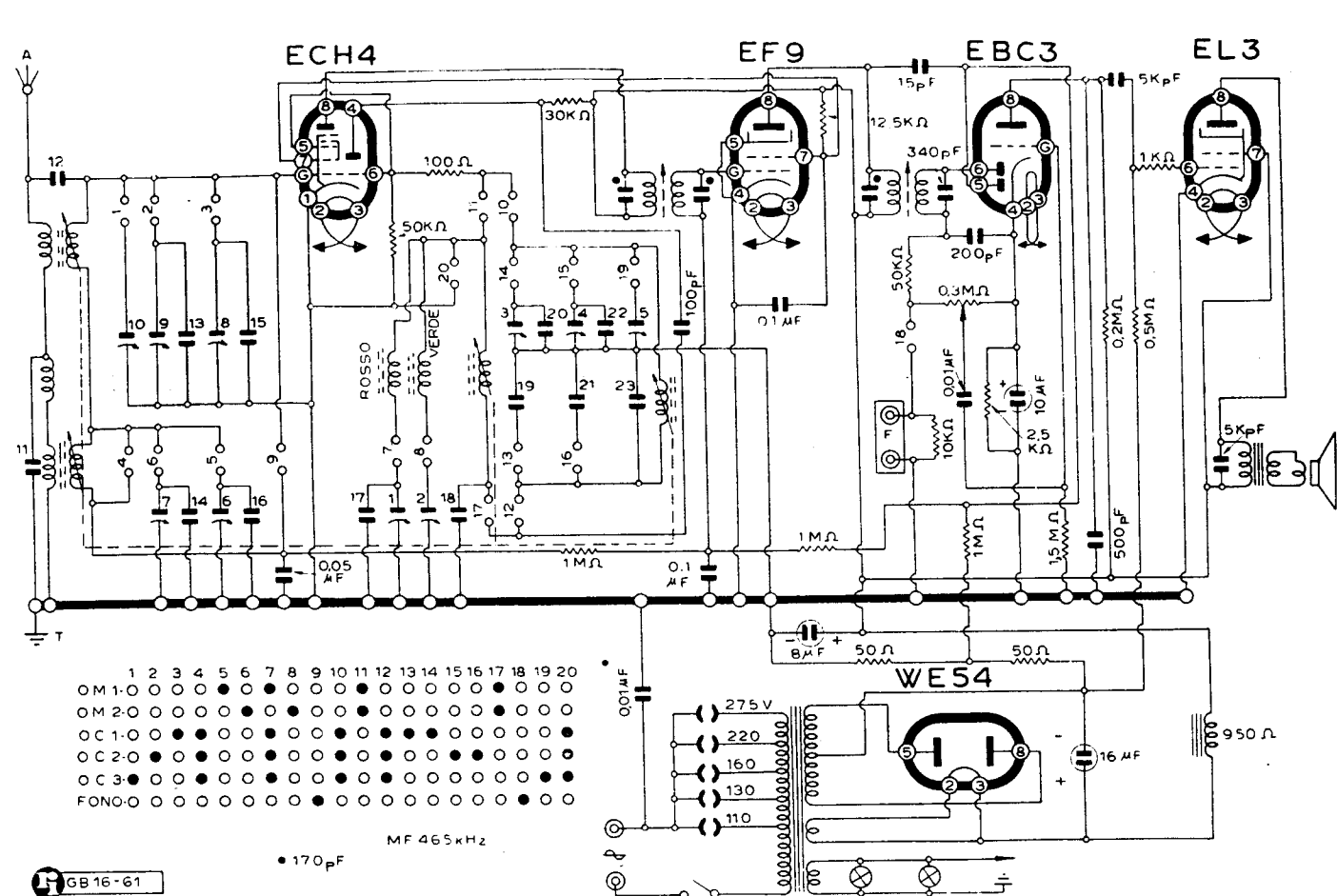
LA VOCE DEL PADRONE - Mod. 1508
