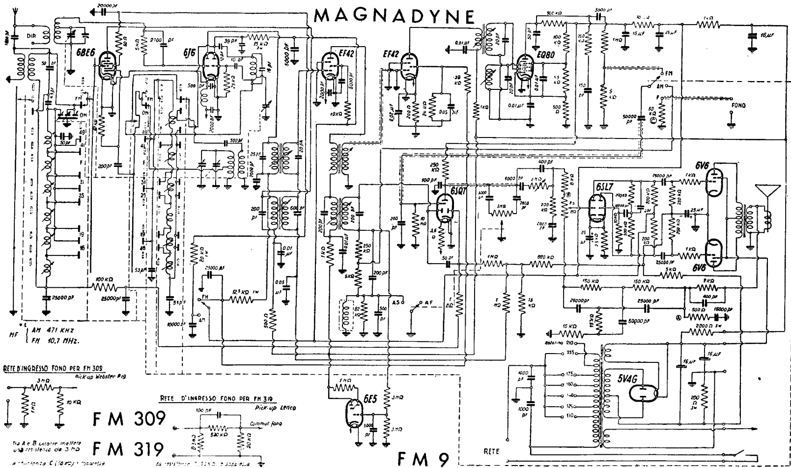
MAGNADYNE RADIO - Mod. FM 9, mod. FM 309 e mod. 319. Ricevitore a modulazione d'ampiezza e a modulazione di frequenza con amplificazione finale in controfase. Una gamma onde medie, sei bande allargate ad onde corte e cortissime e il canale FM a onde ultracorte. Media frequenza AM di 471 kc/s e media frequenza FM di 10,7 Mc/s. Discriminatore FM con enneodo EQ80.
