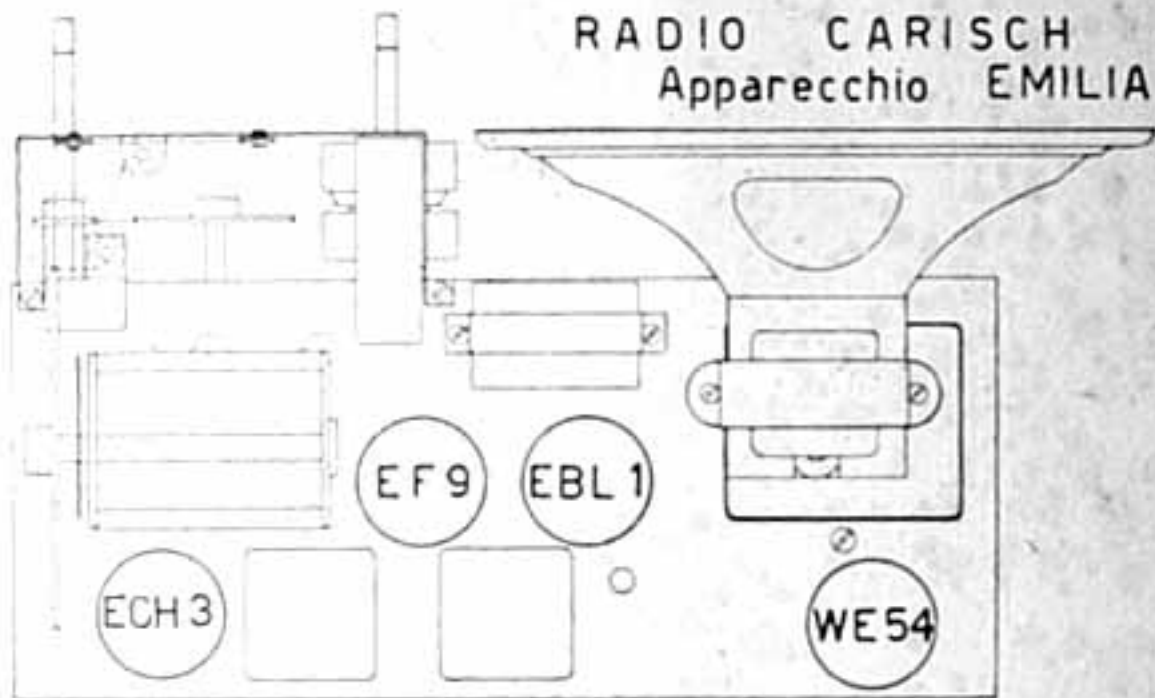
Disposizione valvole
